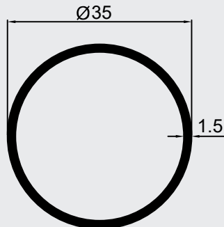
GLS-2499 KG:0.429
