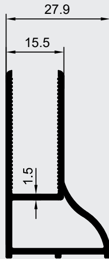
GLS-3027 KG:0.594
