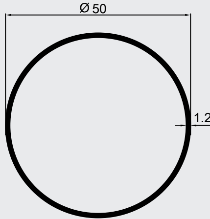
GLS-2500 KG:0.499
