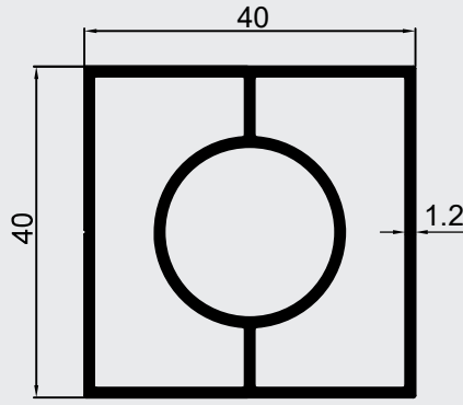
GLS-2562 KG:0.775
