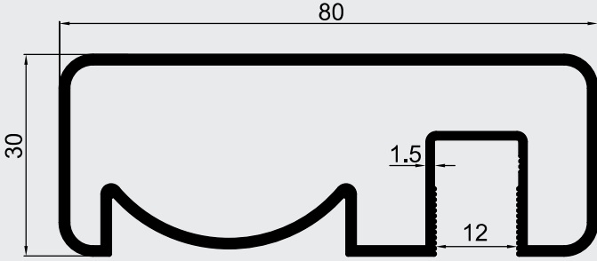
GLS-3003 KG:1.041
