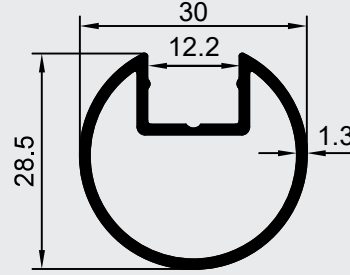
GLS-3019 KG:0.379
