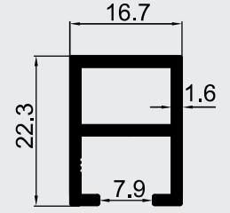
GLS-3002 KG:0.339
