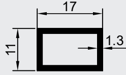
GLS-3020 KG:0.179
