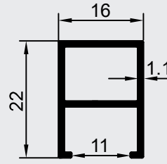
GLS-3021 KG:0.222
