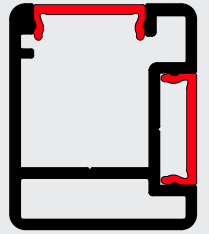
GLS-3016
