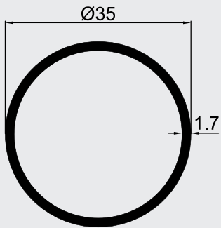
GLS-2436 KG:0.483
