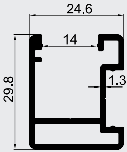
GLS-3016 KG:0.431
