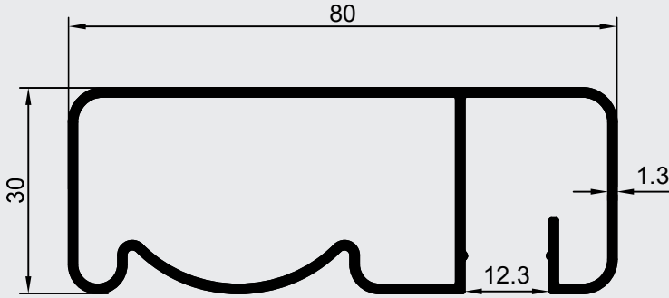
GLS-3023 KG:0.862
