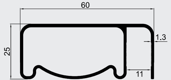
GLS-3011 KG:0.664
